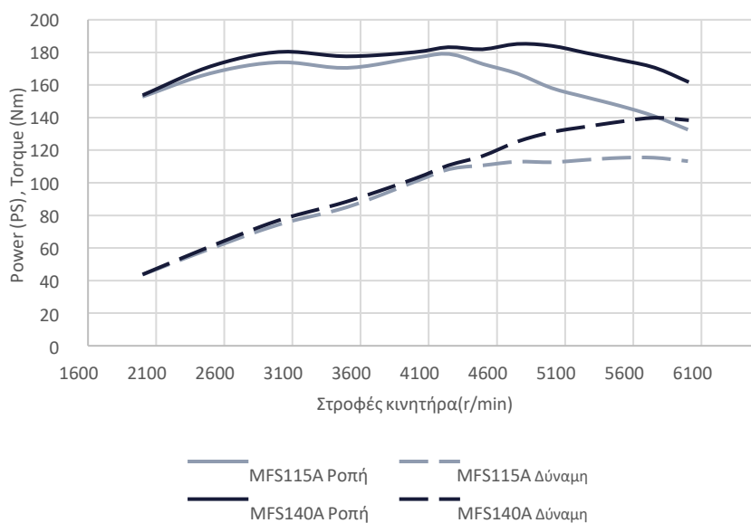
Καμπύλη ισχύος
